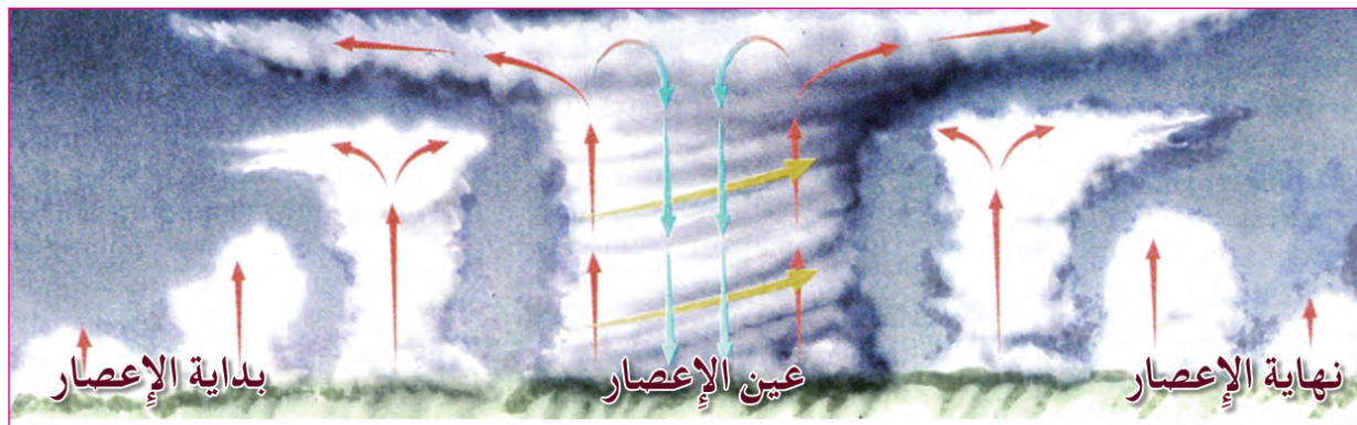
الشكل (١٦): رسم تخطيطي لكيفية حدوث الأعاصير
